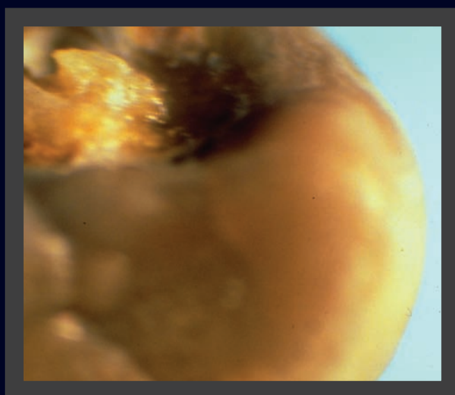
Calcium oxalate monohydrate/apatite
